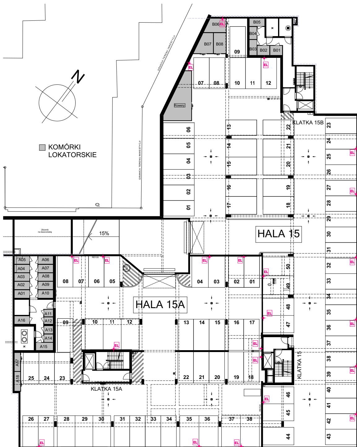
RZUT KONDYGNACJI PODZIEMNEJ
